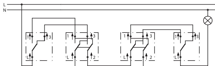
Dwa łączniki krzyżowe w układzie z dwoma łącznikami schodowymi (sterowanie z czterech punktów)
