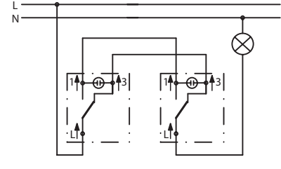
Układ dwóch łączników schodowych podświetlanych
