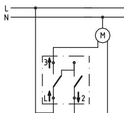
Łącznik żaluzjowy (z blokadą elektryczną równoczesnego załączenia)
