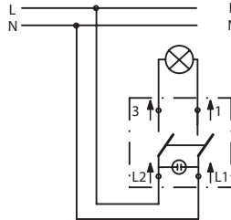
Łącznik dwubiegunowy podświetlany
