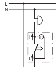
Przycisk dzwonek podświetlany
