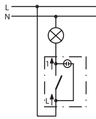
Łącznik jednobiegunowy podświetlany
