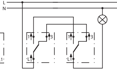
Układ dwóch łączników schodowych
