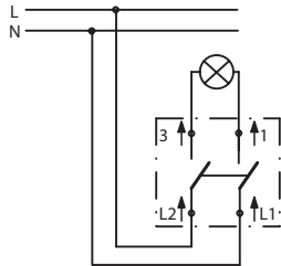
Łącznik dwubiegunowy
