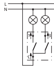
Łącznik świecznikowy
