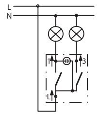
Łącznik świecznikowy podświetlany
