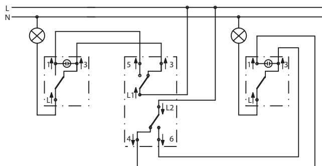
Łącznik podwójny schodowy w układzie z dwoma łącznikami schodowymi
