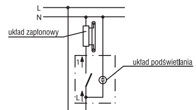
Łącznik jednobiegunowy podświetlany obciążenie świetłówką kompaktową
