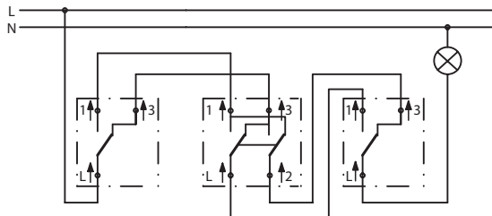
Łącznik krzyżowy w układzie z dwoma łącznikami schodowymi
