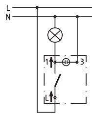
Łącznik jednobiegunowy z sygnalizacją załączenia
