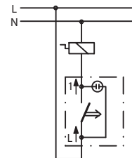
Przycisk światło podświetlany
