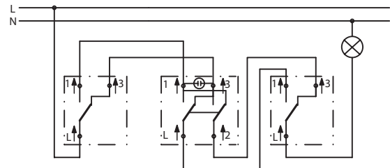
Łącznik krzyżowy podświetlany w układzie z dwoma łącznikami schodowymi
