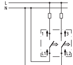
Przycisk podwójny
